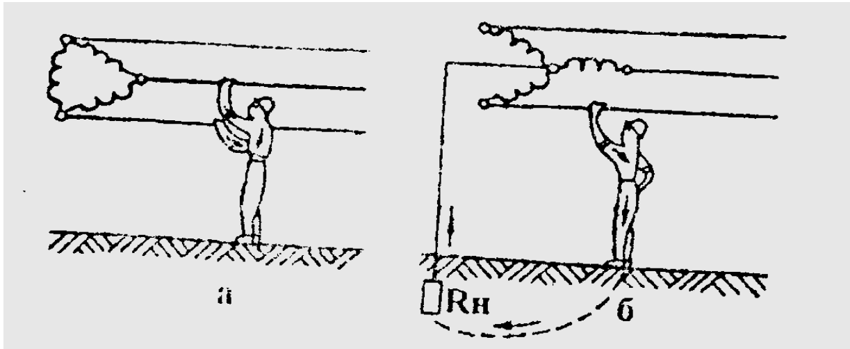
Рис.1 Схемы включения человека в электросеть: а – двухфазная; б – однофазная к сети с глухозаземленной нейтралью.
